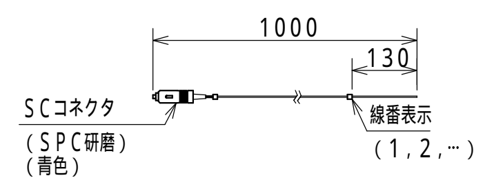
片端光コネクタ付心線 (R15対応) SM (8.6/125)
