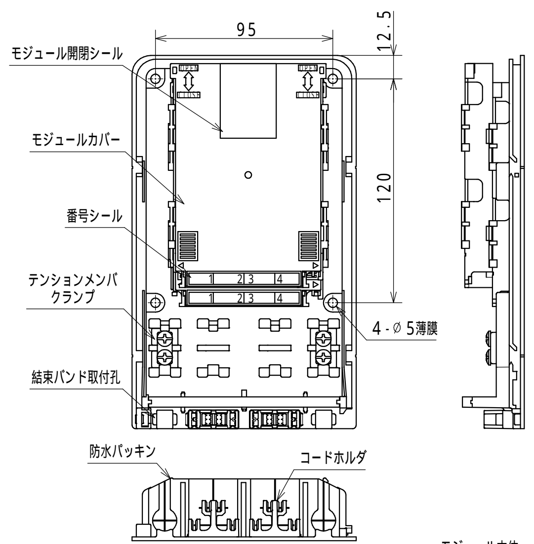
内部詳細図
