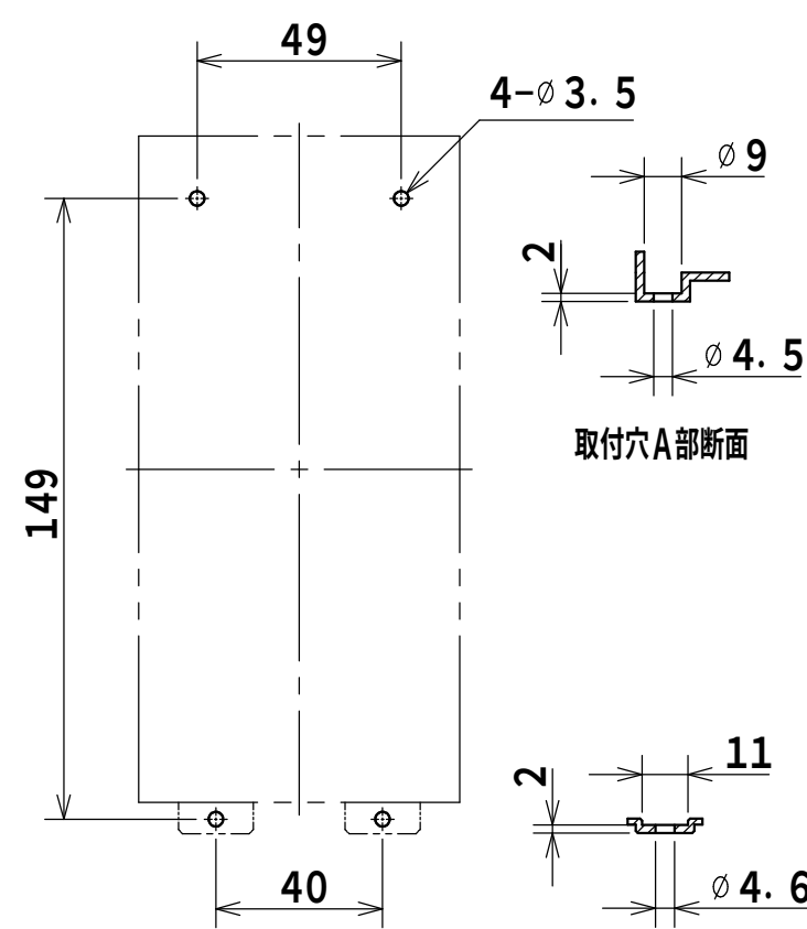
取付穴寸法
