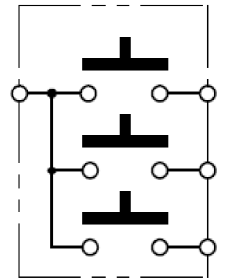
内部回路図
