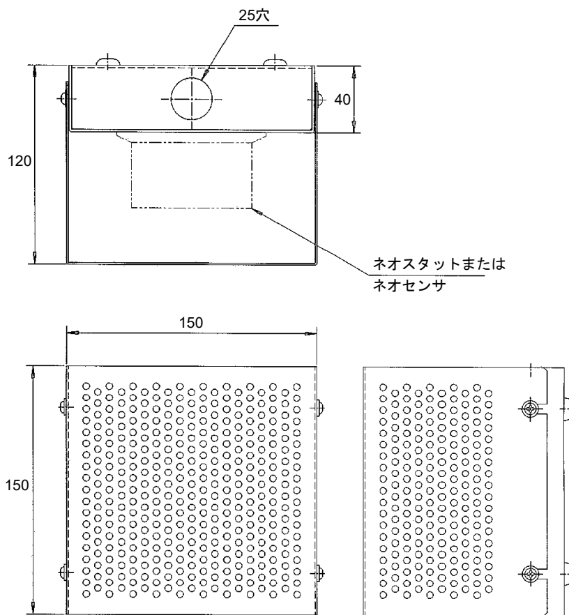
外形寸法図 (mm)
