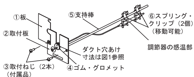
図2 取付図
