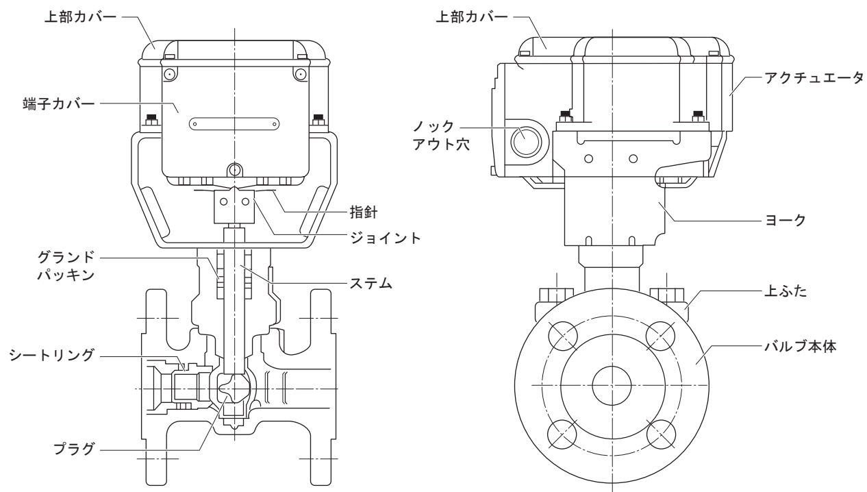
図3 各部の名称
