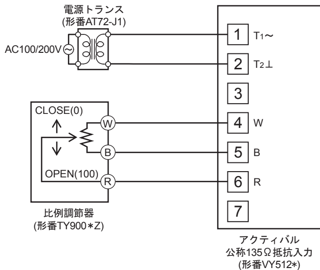
図 15 ネオスタットとの接続例
