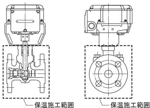
図6 保温施工
