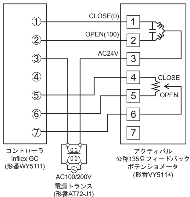
図 14 Inflex GC との接続例
