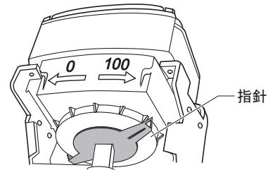
図7 工場出荷時の指針位置
