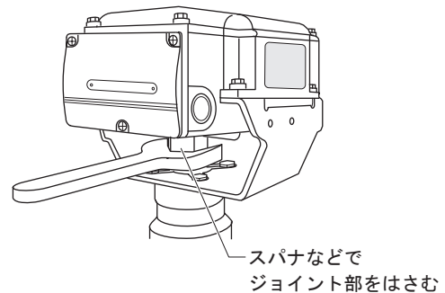
図8 手動開閉操作
