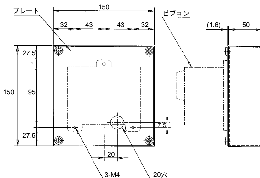
裏面図
