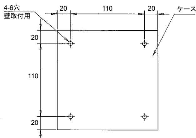
裏面図
