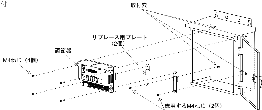
図8 防雨ケース取付(既設/上側)
