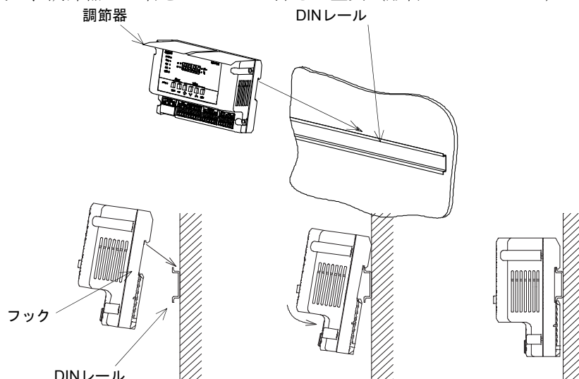
図10 DINレール取付
