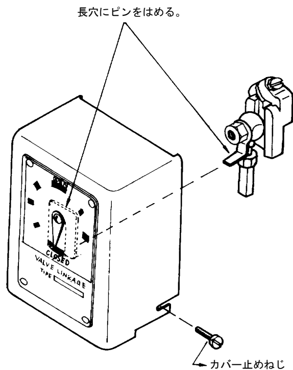
図11 ピンの取付
