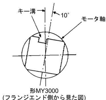
図4 コントロールモータ“閉の位置”
