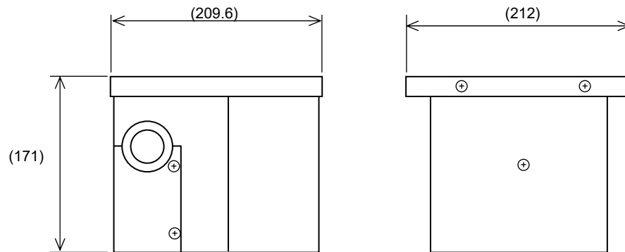
外形寸法図 (mm)
