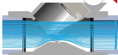
アングルシート構造 JSB Series
