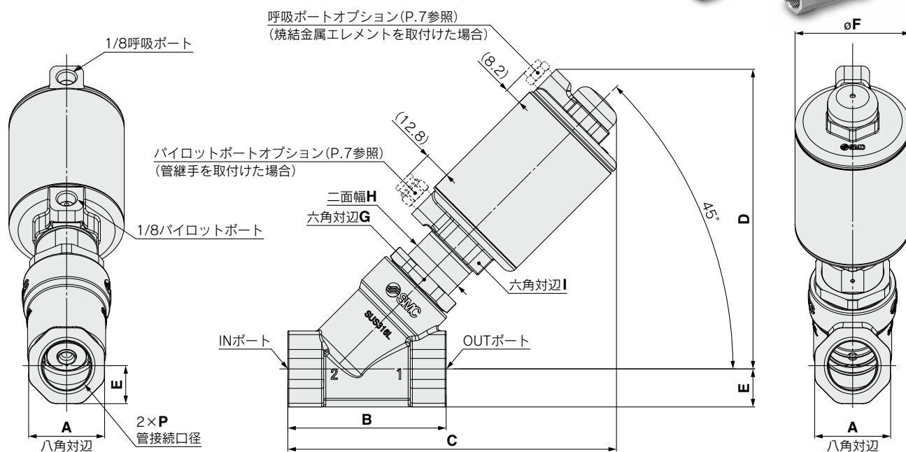
寸法表
