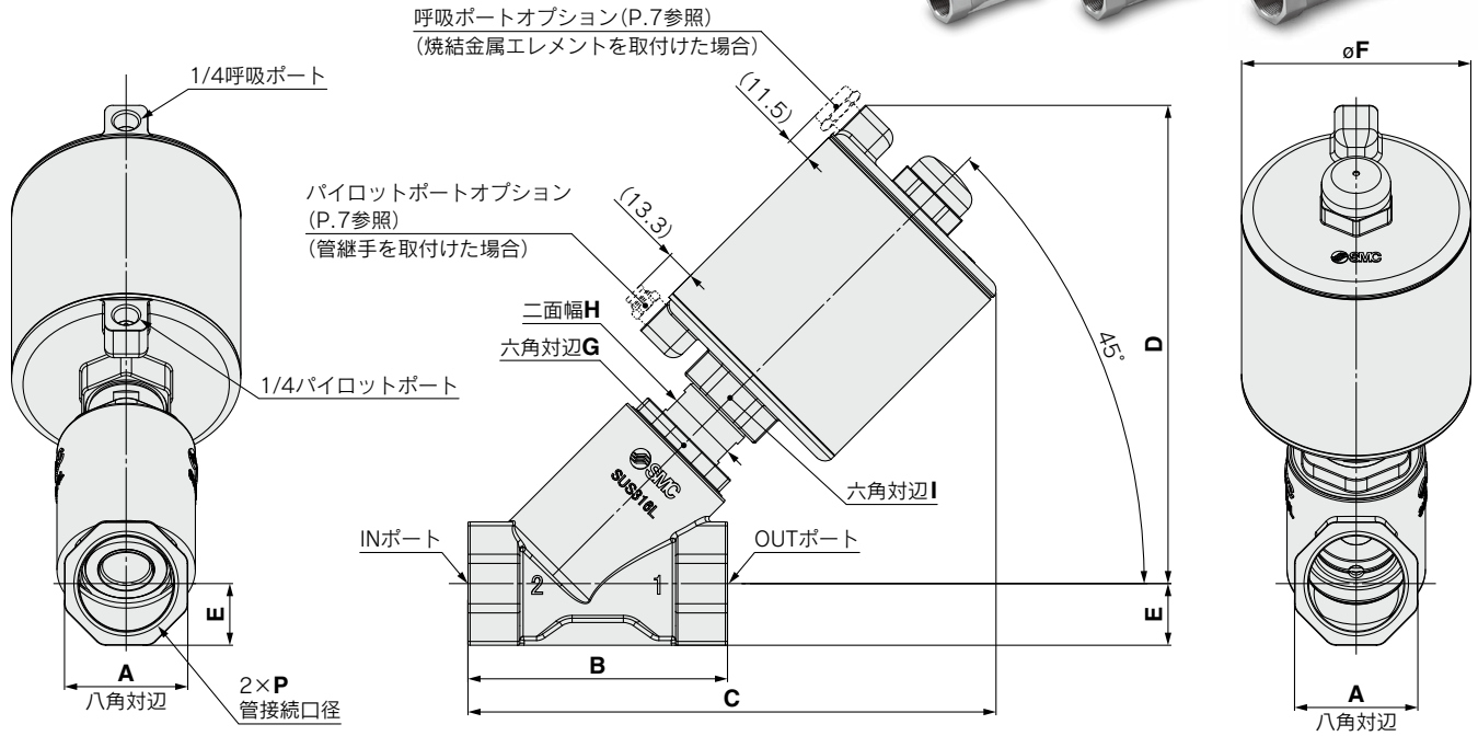
寸法表
