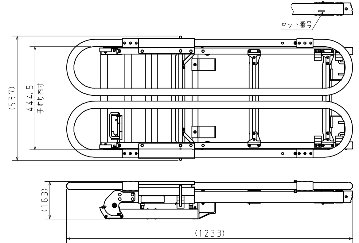
収納状態
