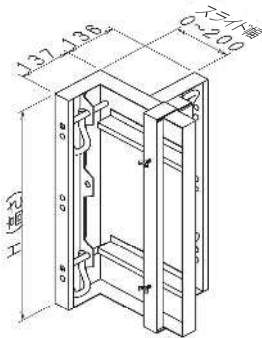
136×0-200×137 スライド段付パネル(天地)
