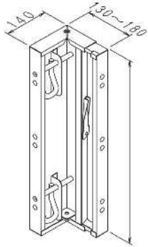
140xワンタッチスライド内コーナー (130-180mm) 止め金具付 天地
