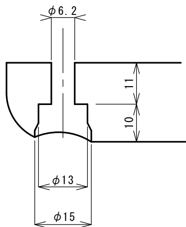
取付用穴寸法
