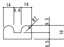
側面B
