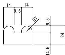
断面A-A'
