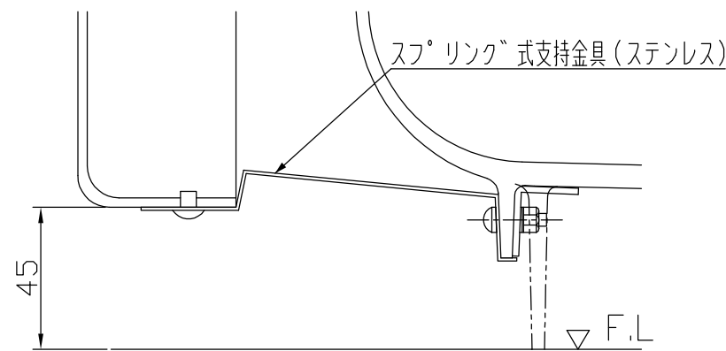
エプロン支持部詳細図
