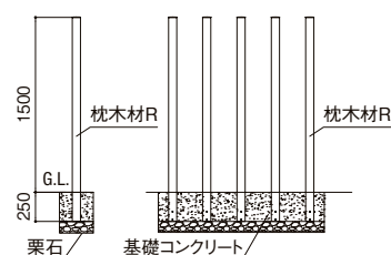
枕木材R 寸法図
