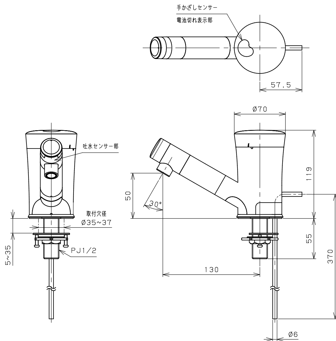
自動水栓 (SS2P-VB)
