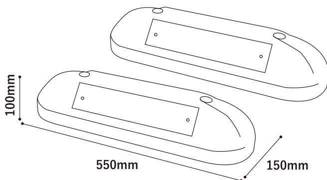
カーストッパー本体×2
