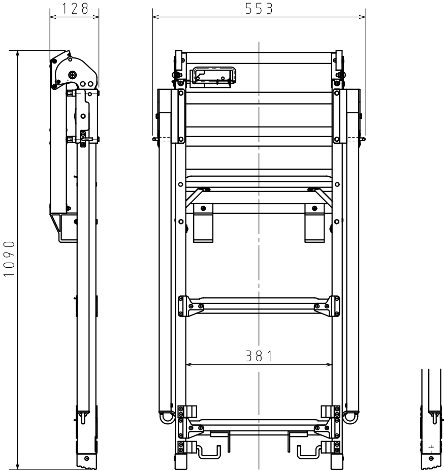
収納状態
