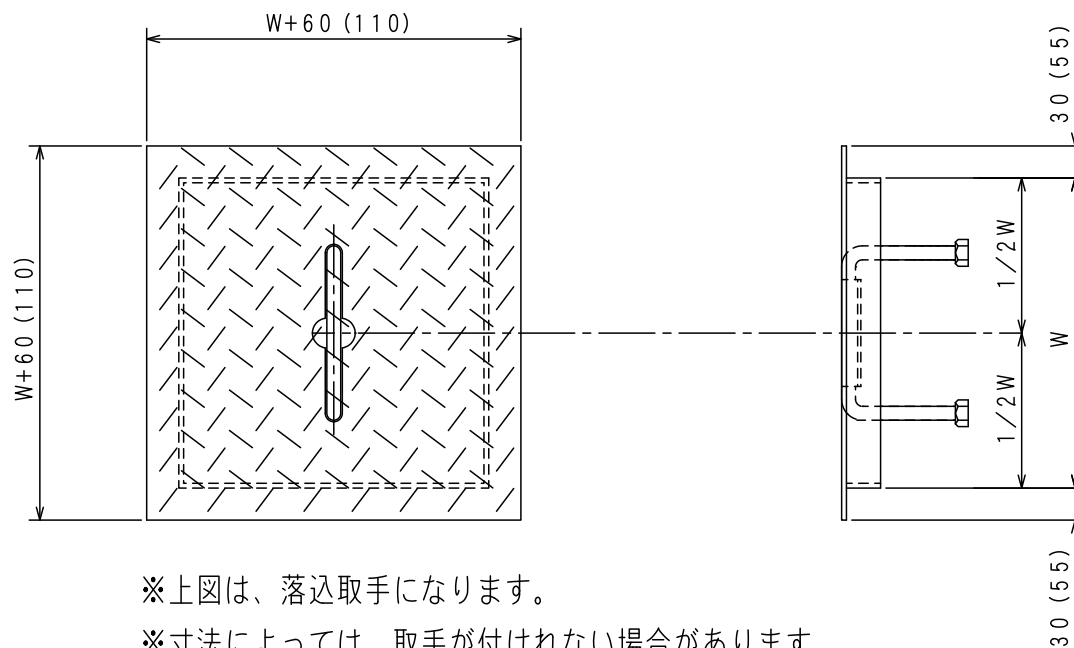
オプション取手 1 個の取付位置 中心の位置
