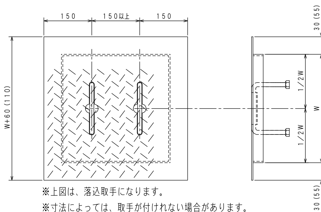
オプション取手 2 個の取付位置 両端部より、150 mm の位置
