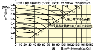
【GL-120型圧力調整器 流量表】
