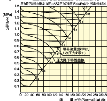
【GL-180型圧力調整器 流量表】
