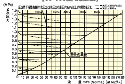
【GS-100型 流量表】
