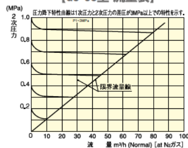
【GS-60型 流量表】
