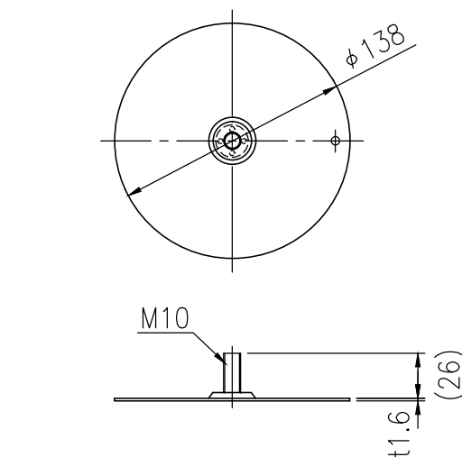
⑧ スチールスペーサー詳細図 S=1/4
