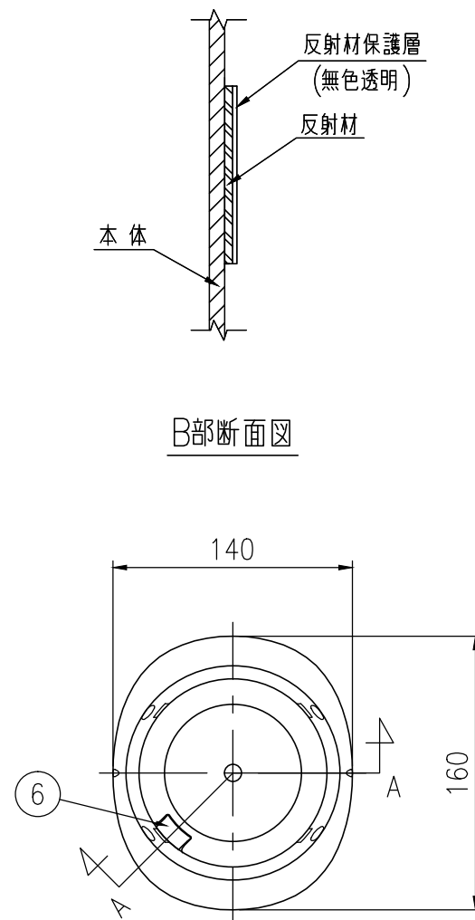
平面図 S=1/4
