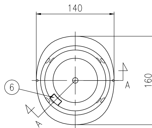
平面図 S=1/4
