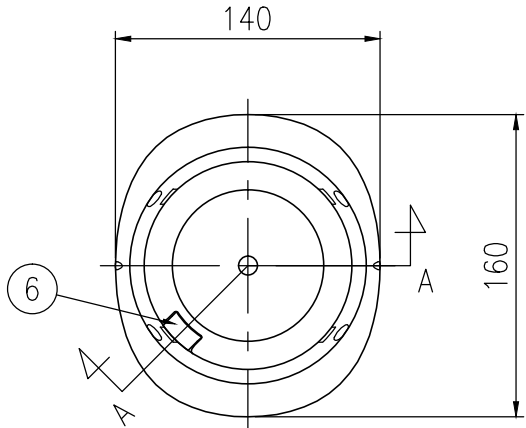
平面図 S=1/4
