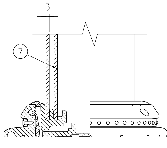
B部断面図
