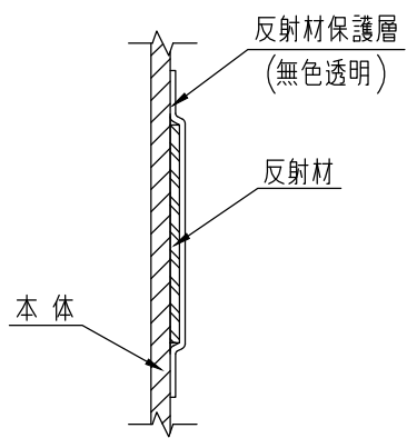
B部断面図
