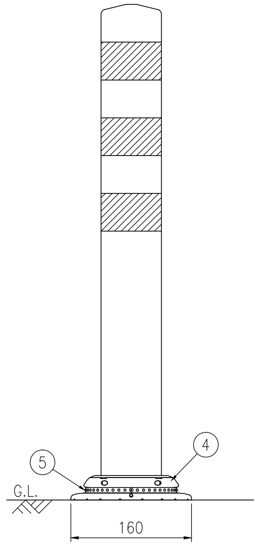
設置図 S=1/5
