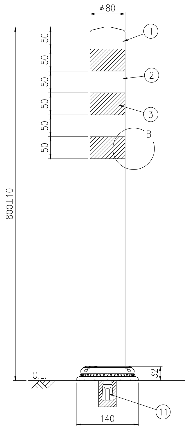
設置図 S=1/5
