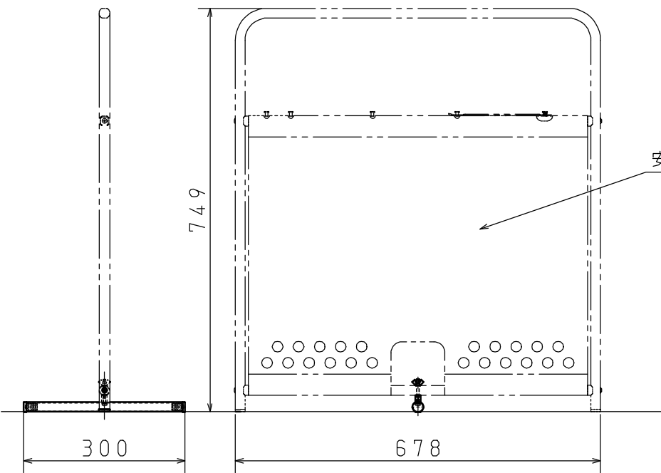
使用時 (S = 1 : 10)
