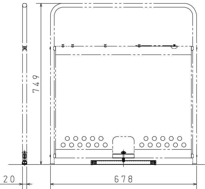
収納時 (S = 1 : 10)
