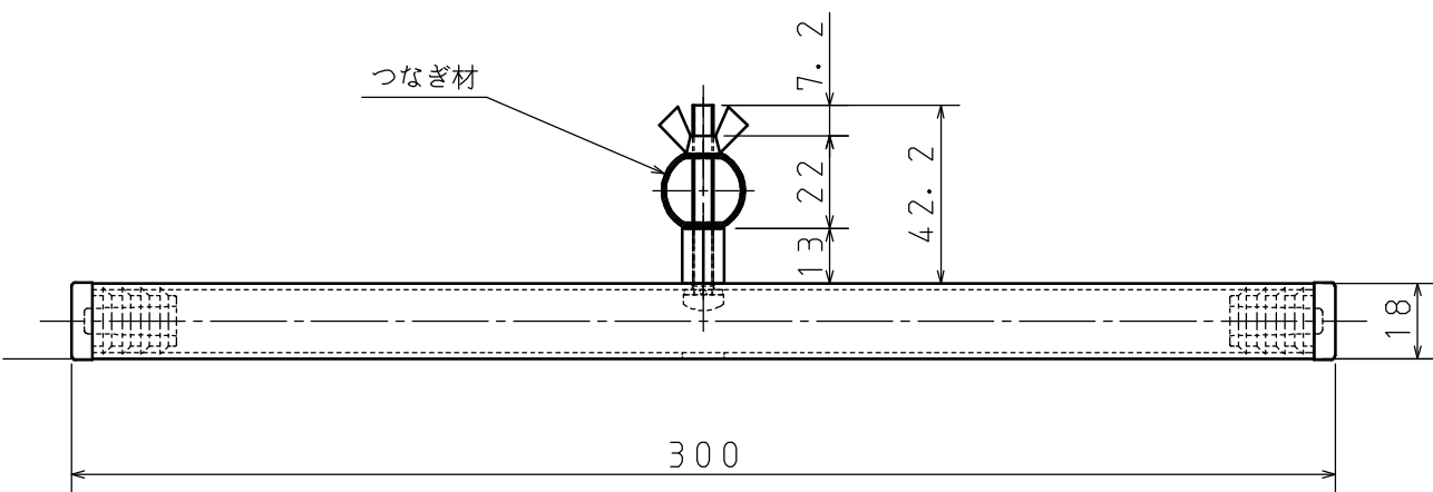
A-A断面
