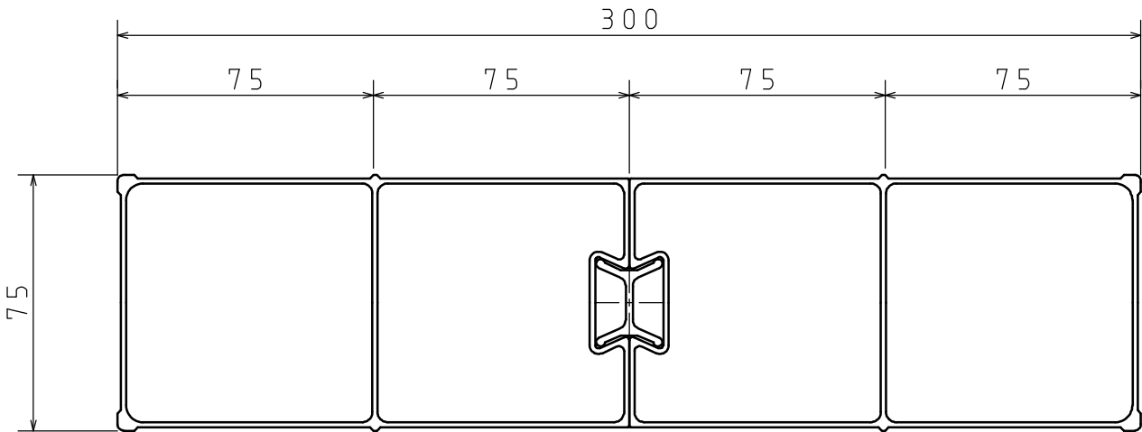
足場板断面詳細
