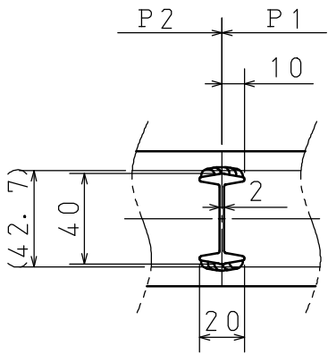
B 矢視図 (S = 1 : 3)
