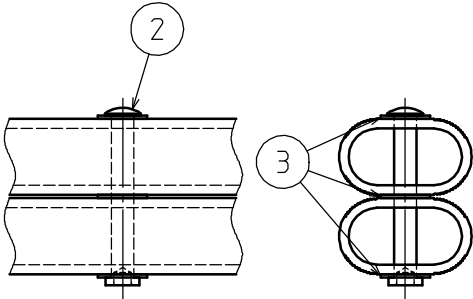
矢視A-A (S=1:2)
