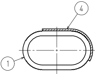
矢視B-B (S=1:1)
