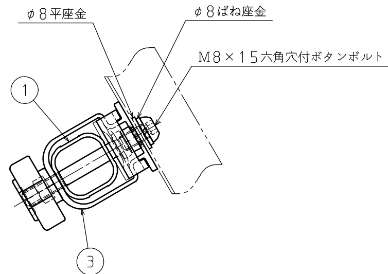
A-A矢視
