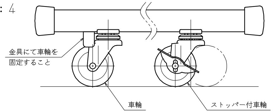
ATL-1WA収納状態図
