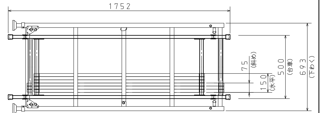
ATL-2WA収納状態図
