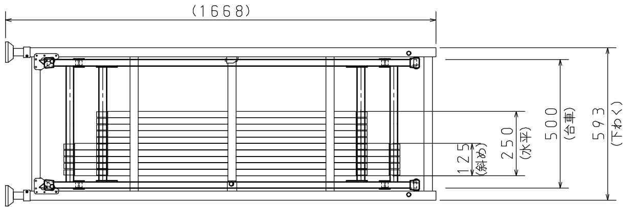
ATL-3A収納状態図
