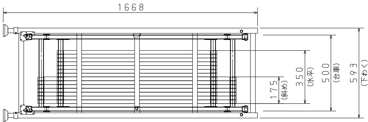
ATL-3A収納状態図
