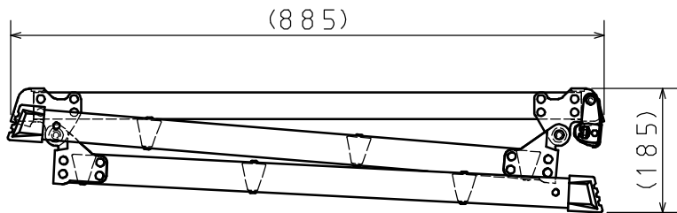
収納状態図
