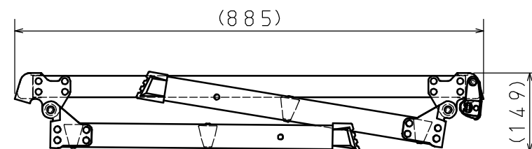
収納状態図
