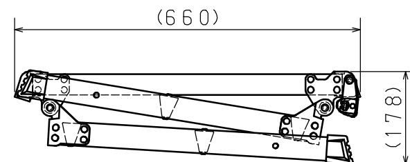
収納状態図
