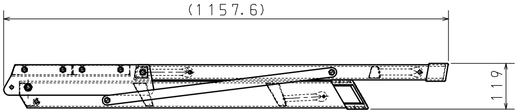
収納状態図
