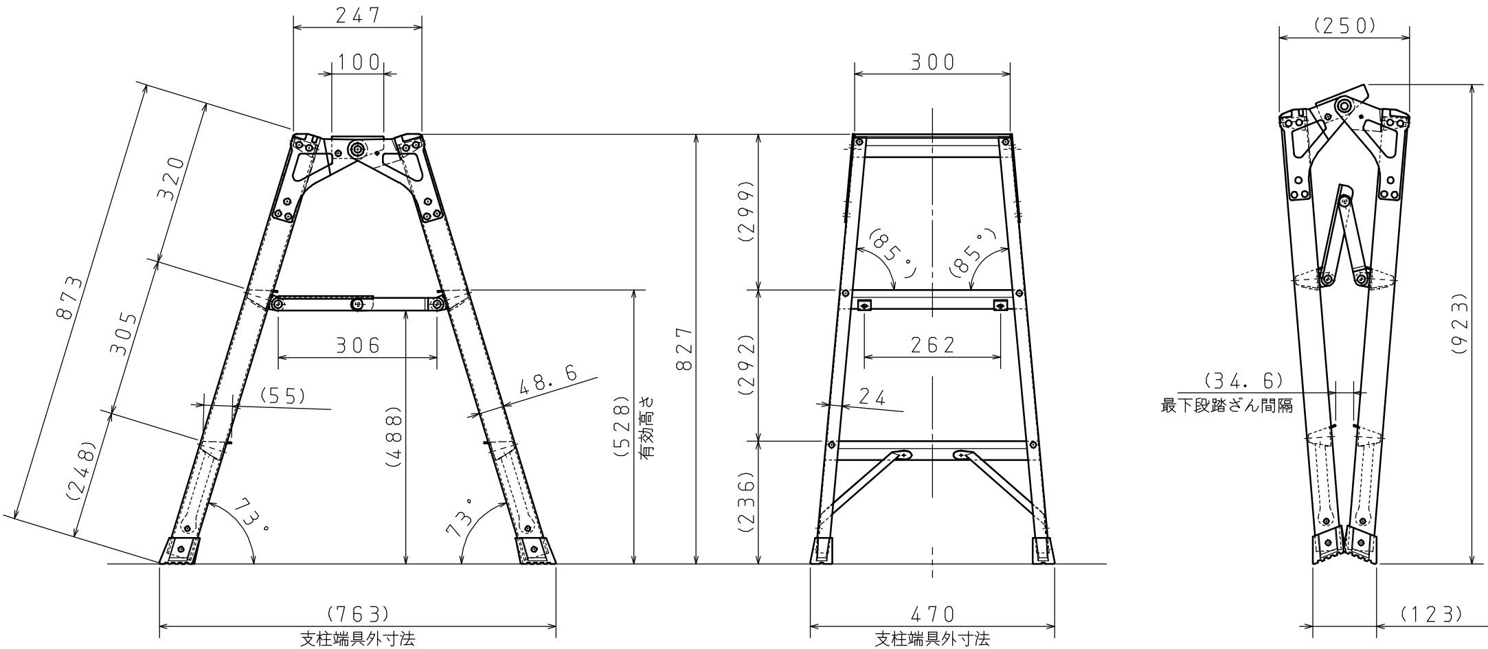
収納状態図
