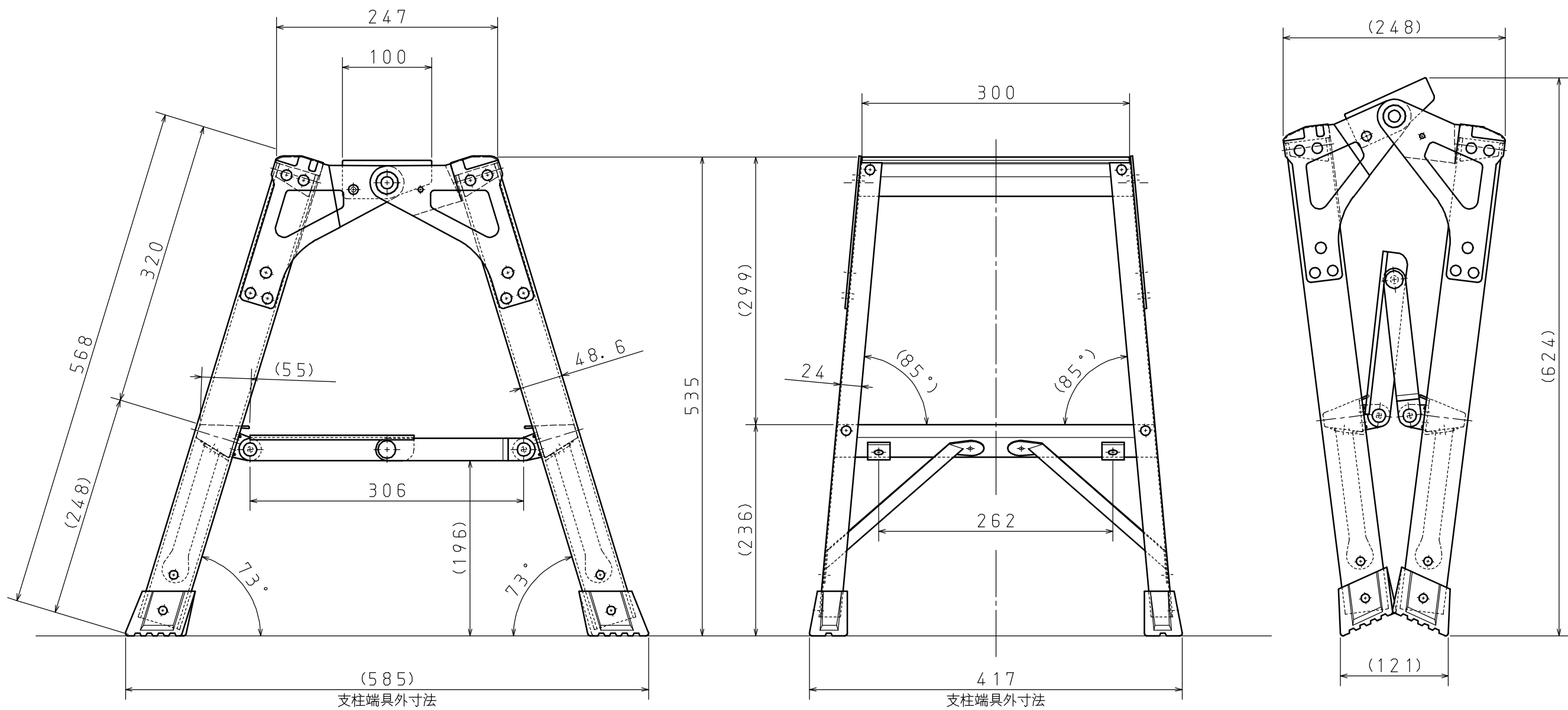
収納状態図
