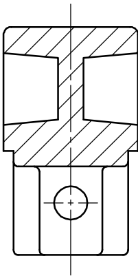
A-A断面
