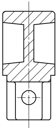
A-A断面
