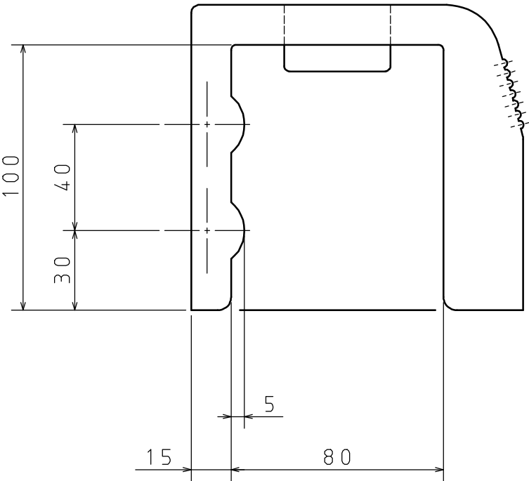
断面A-A
