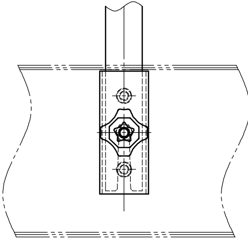
ソケット取付け詳細図 S = 1 : 3
