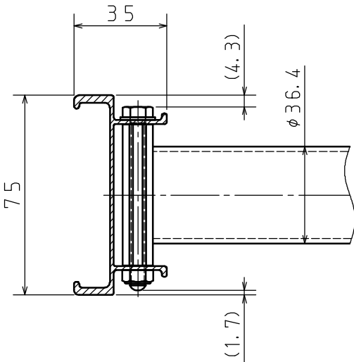
A-A断面 S = 1 : 2
