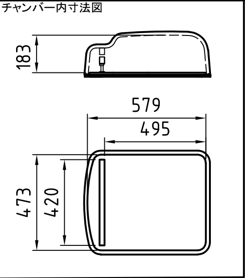
チャンバー内寸法図
